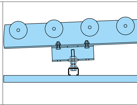
Højdejusterbar gulvbjælke
