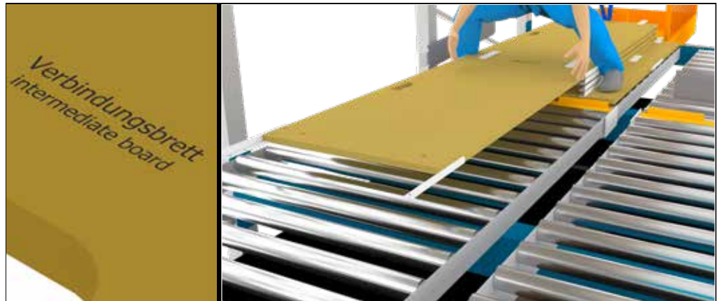
På billedet 34: Udlægning af forbindelsesplader
