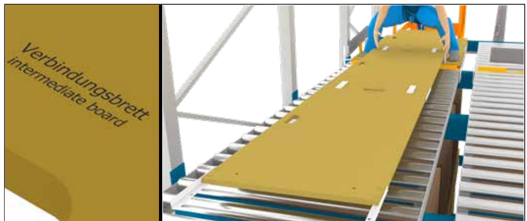
På billedet 35: Udlægning af forbindelsesplader
