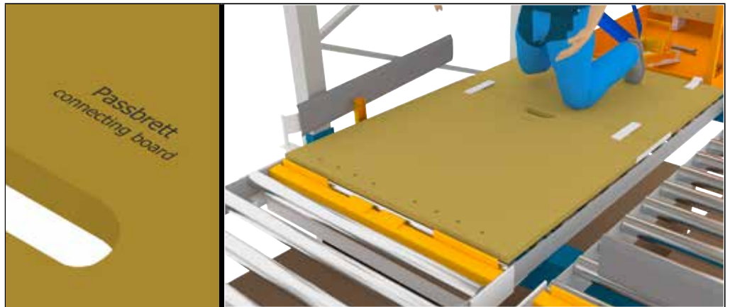
På billedet 32: Forbindelse af passagebrættet til startbrættet
