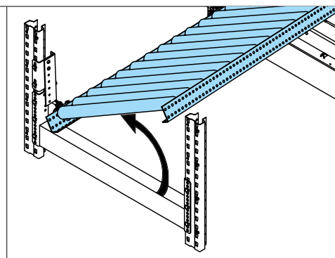
Opklappelig rullebane
